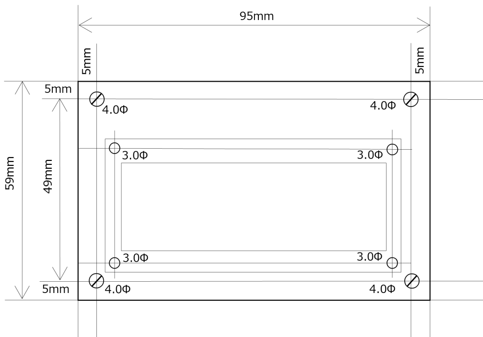
上面図 (アクリル)
