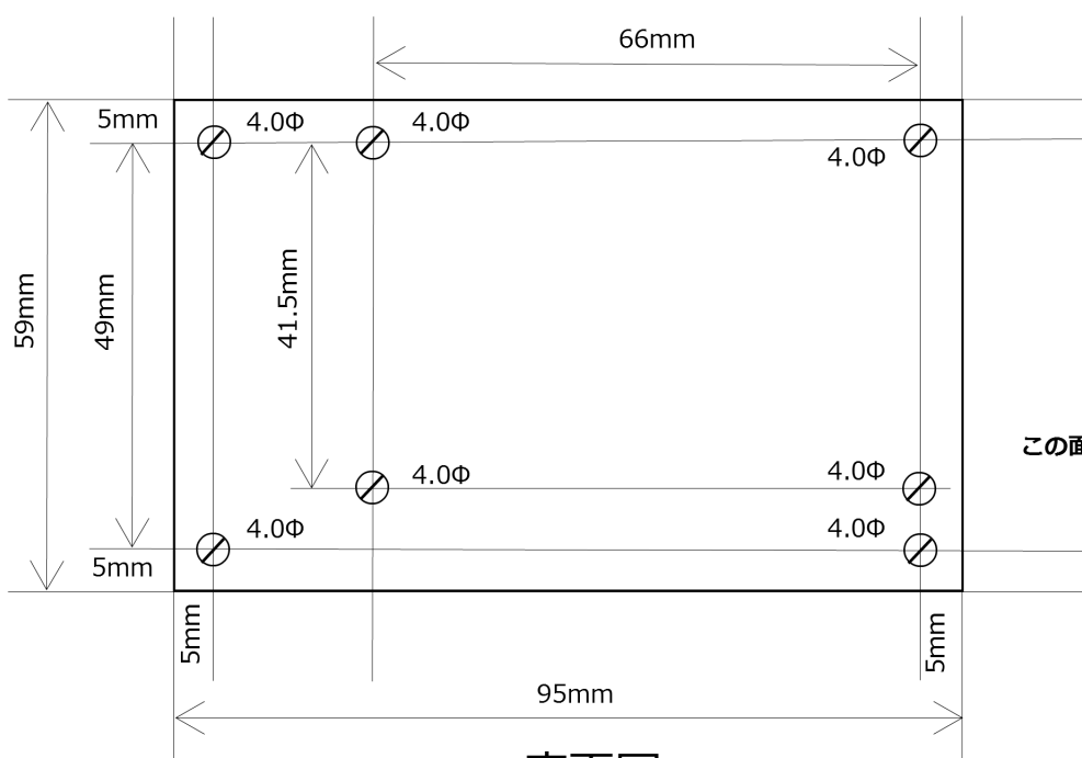
底面図 (上から見た図)
