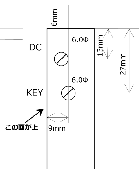
側面図 (右)
